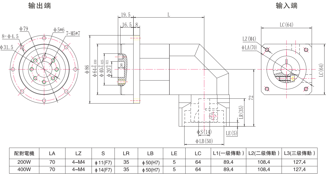
KDR60外形图
