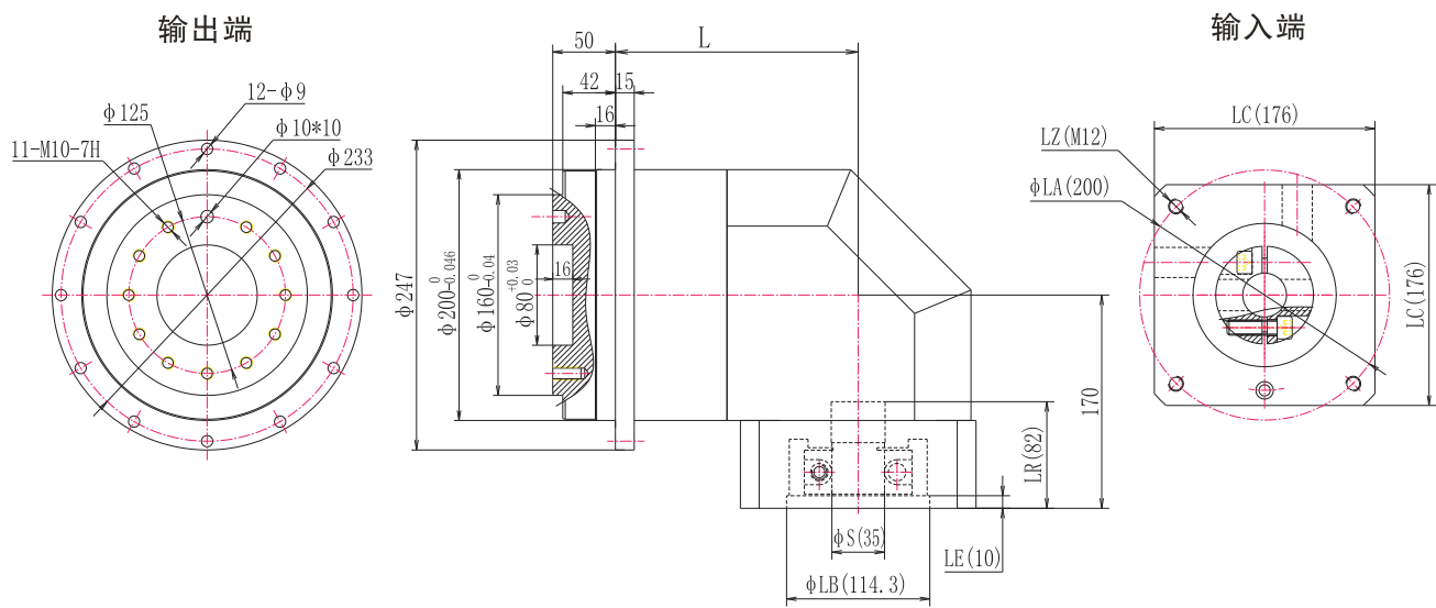
KDR200外形图
