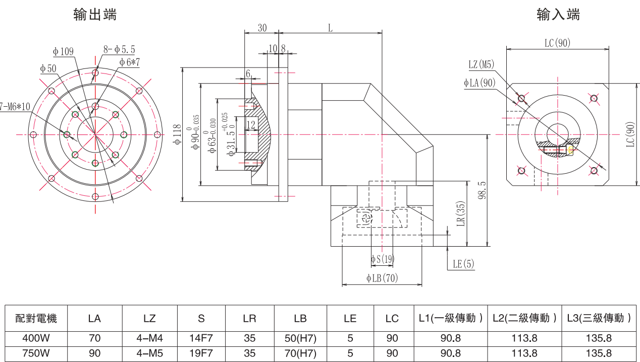
KDR90外形图
